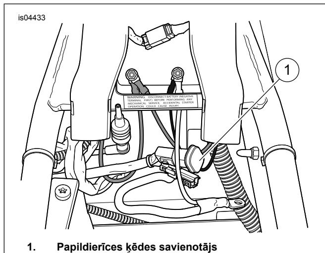
Attēls 4 Papildierīces ķēdes savienotājs
