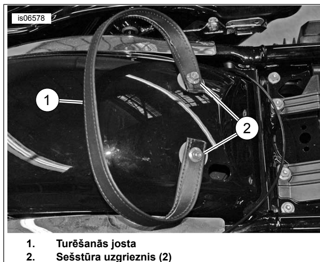
Attēls 3 Satveršanas siksnas uzstādīšana
