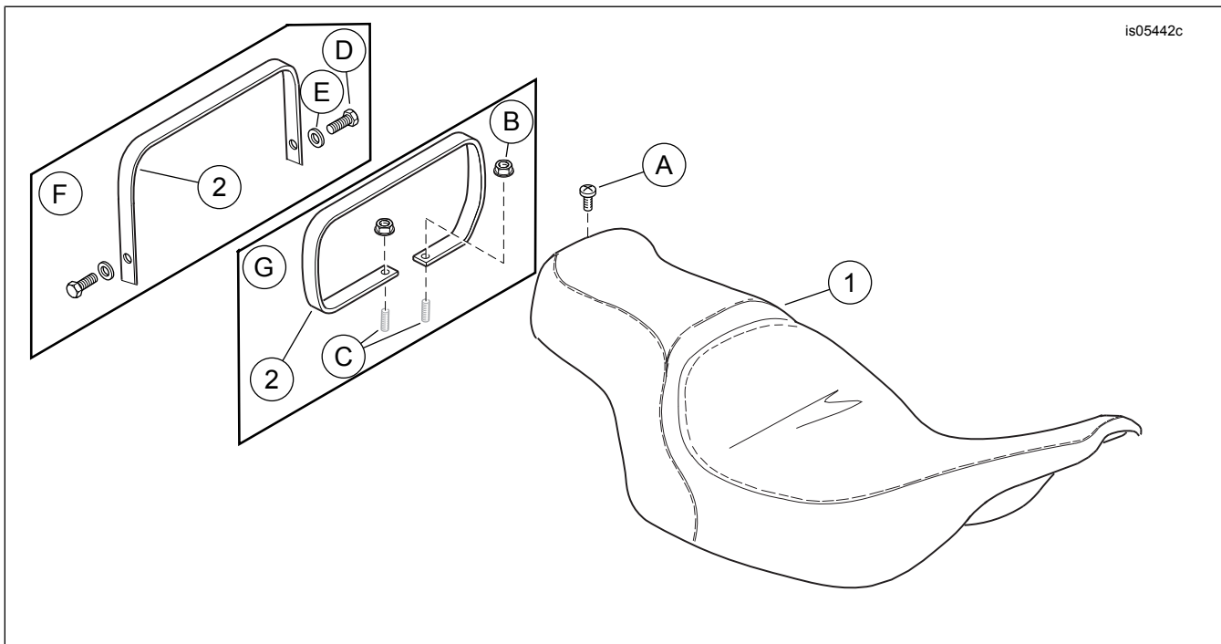
Attēls 7 Apkopes daļas: Apsildāms sēdekļs
