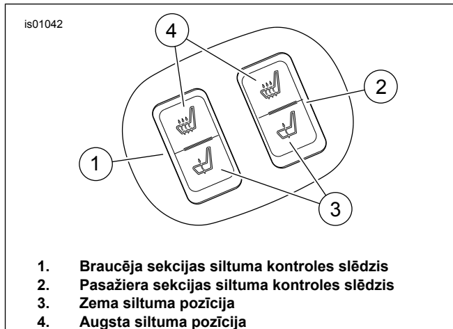
Attēls 6 Sēdekļa apsildes vadības slēdži
