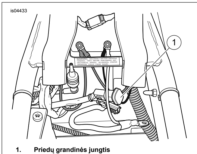
Pav 4. Priedų grandinės jungtis
