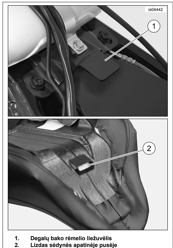
Pav 5. Sėdynės priekinės dalies montavimas
