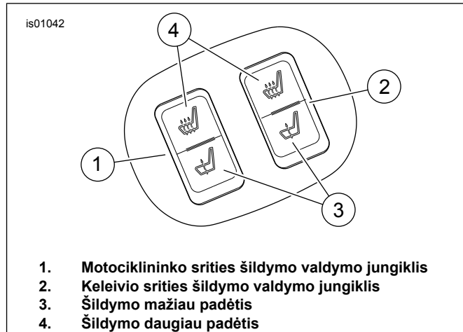
Pav. 6. Sėdynių šildymo valdymo jungikliai
