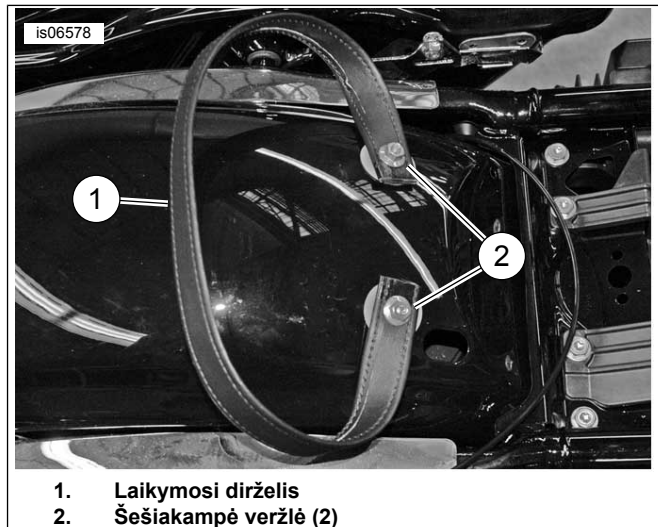
Pav 3. Laikymosi dirželio montavimas
