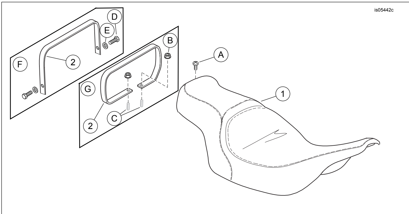
Pav. 7. Dalys, reikalingos užduočiai atlikti Šildomoji sėdynė
