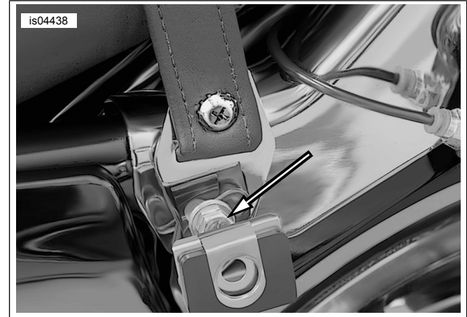
Pav 1. Keleivio laikymosi dirželio nuėmimas (pavaizduotas 2008 m. modelis)
