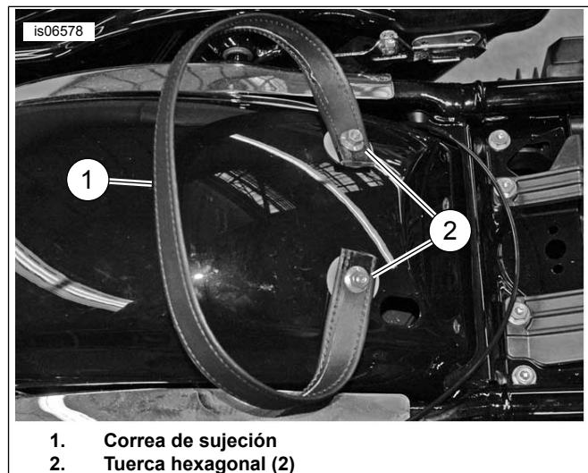
Figura 3. Instalación de la correa de sujeción
