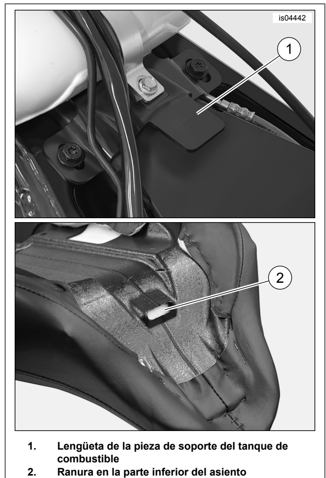
Figura 5. Montaje del asiento delantero
