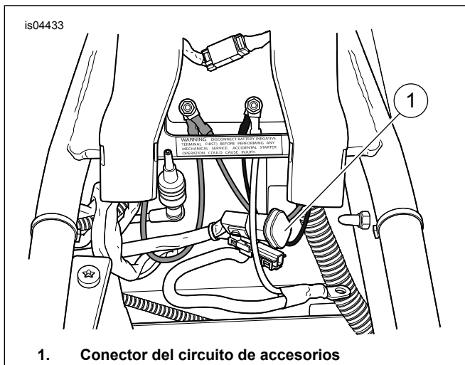
Figura 4. Conector del circuito de accesorios
