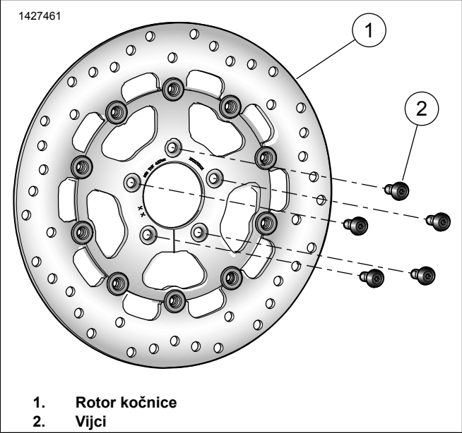
Slika 1. Servisni dijelovi: Kompleti rotora (diska) prednje kočnice
