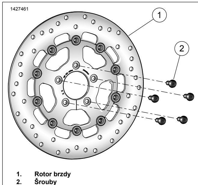
Ilustrace 1. Servisní díly: Sady předních brzdových kotoučů
