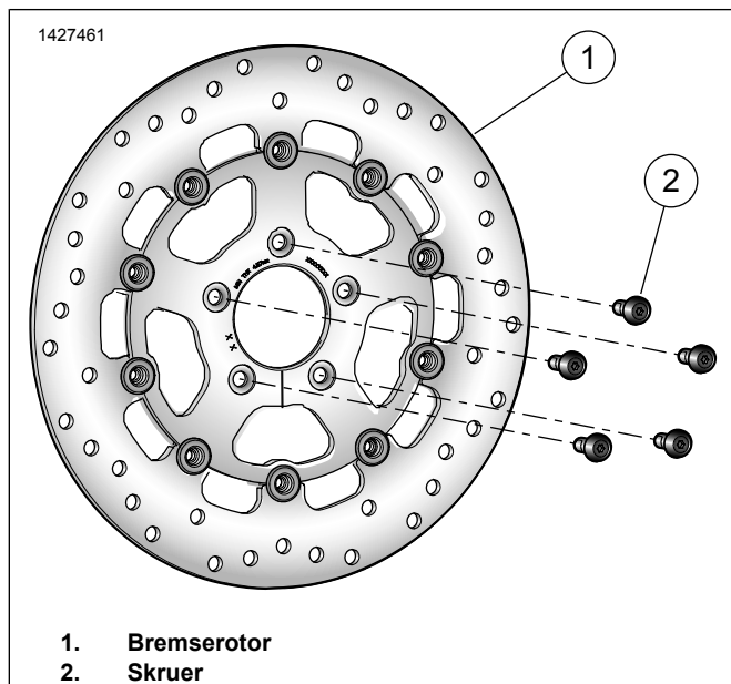
Figur 1. Reservedele: Forbremserotorsæt (skive)
