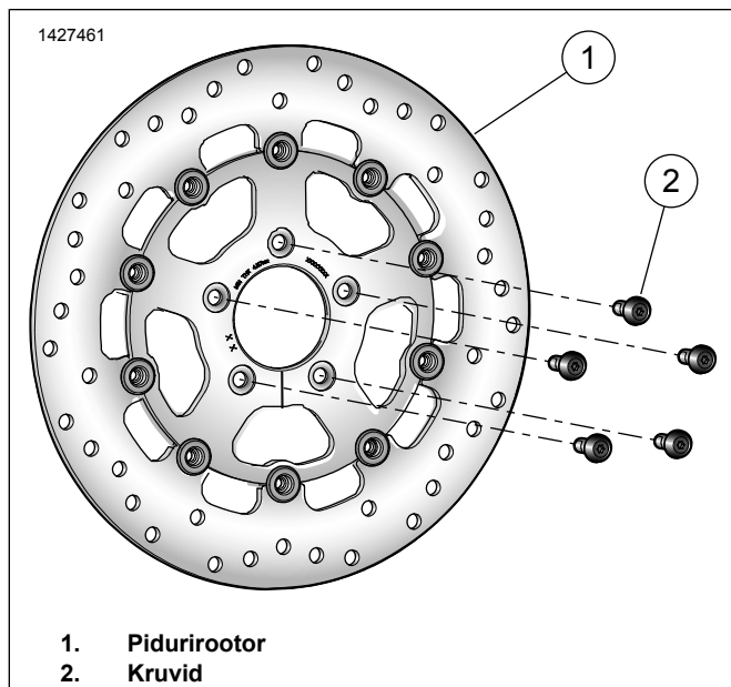
Joonis 1. Hoodatavad osad: Eesmise pidurirootori (ketta) komplekt
