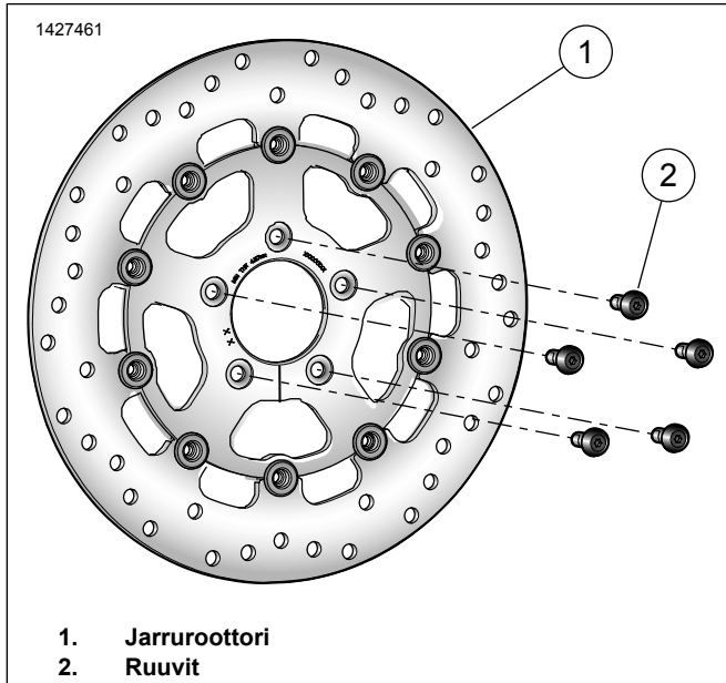
Kuva 1. Huolto-osat: Etujarruroottorin levysarja
