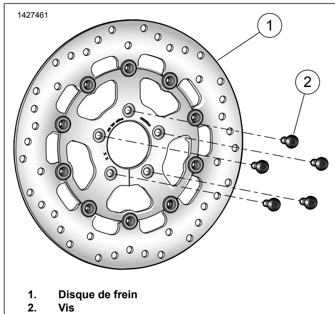
Figure 1. Pièces de rechange : Kits de disque de frein avant (disque)
