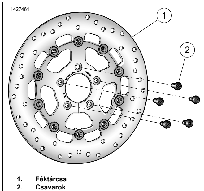
Ábra 1. Szervizelhető alkatrészek: Első féktárcsa készlet
