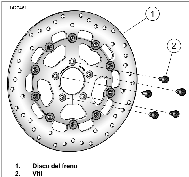
Figura 1. Parti di ricambio: Kit disco del freno anteriore
