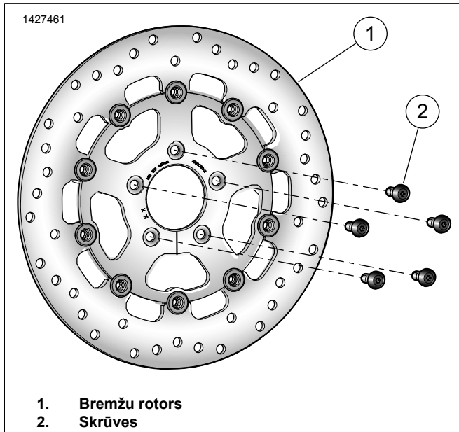
Attēls 1 Apkopes daļas: Priekšējo bremžu rotora (diska) komplekti
