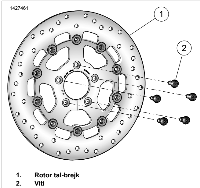
Figura 1. Parts tas-Service: KITS TAR-ROTOR (DISC) TAL-BREJK TA' QUDDIEM
