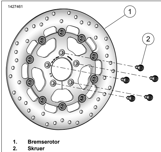
Figur 1. Servicedeler: Sett for fremre bremserotor
