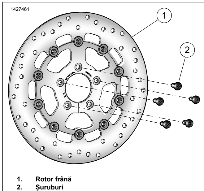
Figura 1. Componente de service: Kit-uri Rotor (Disc) frână față
