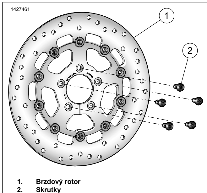
Obrázok 1. Servisné diely: Súpravy predných brzdových kotúčov
