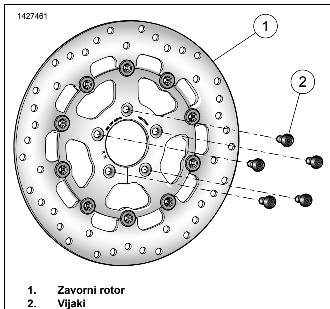
Slika 1. Servisni deli: Kompleti sprednjega zavornega rotorja (diska)
