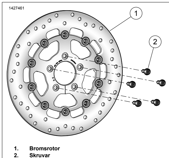
Figur 1. Reservdelar: Frambromsrotorsatser (skivor)
