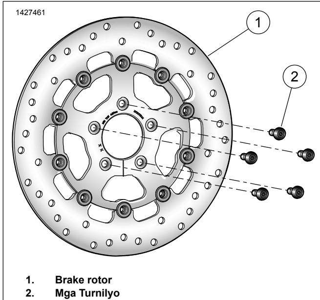
Figure 1. Mga Pamalit na Piyesa: Mga Kit ng Brake Rotor (Disc) sa Harap
