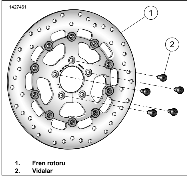
Şekil 1. Servis Parçaları: Ön Fren Rotoru (Diski) Kitleri
