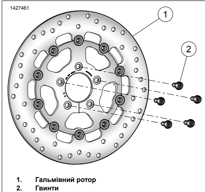
Малюнок 1. Запчастини, що обслуговуються: Комплекти (дискового) ротора переднього гальма
