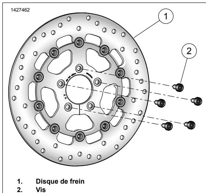
Figure 1. Pièces de rechange : Kits de disque de frein arrière
