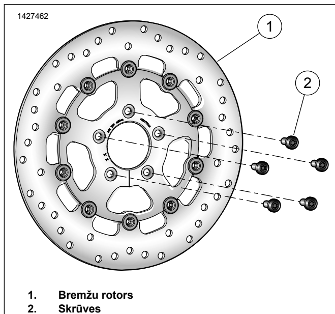
Attēls 1 Apkopes daļas: Aizmugurējā bremžu rotora (diska) komplekti
