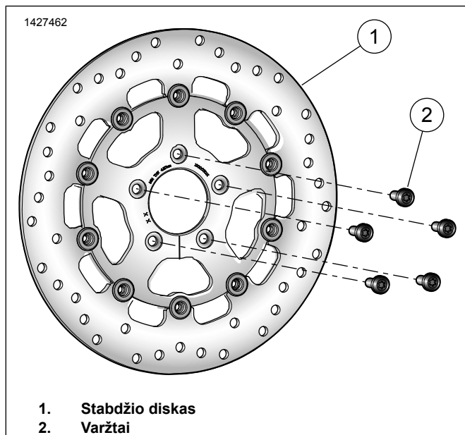
Pav 1. Dalys, reikalingos užduočiai atlikti Užpakalinio stabdžio diskų komplektai
