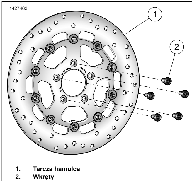
Rysunek 1. Elementy zestawu serwisowego: Zestawy tarczy hamulca tylnego (tarcza)
