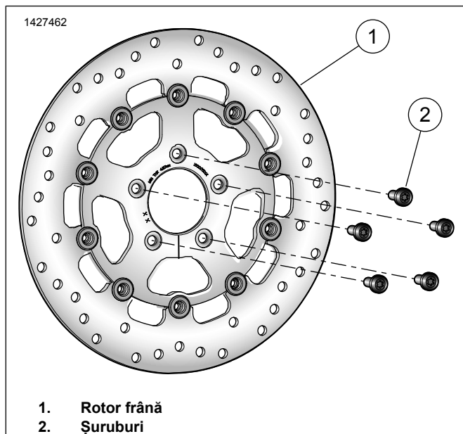
Figura 1. Componente de service: Kit-uri rotor (disc) frână spate
