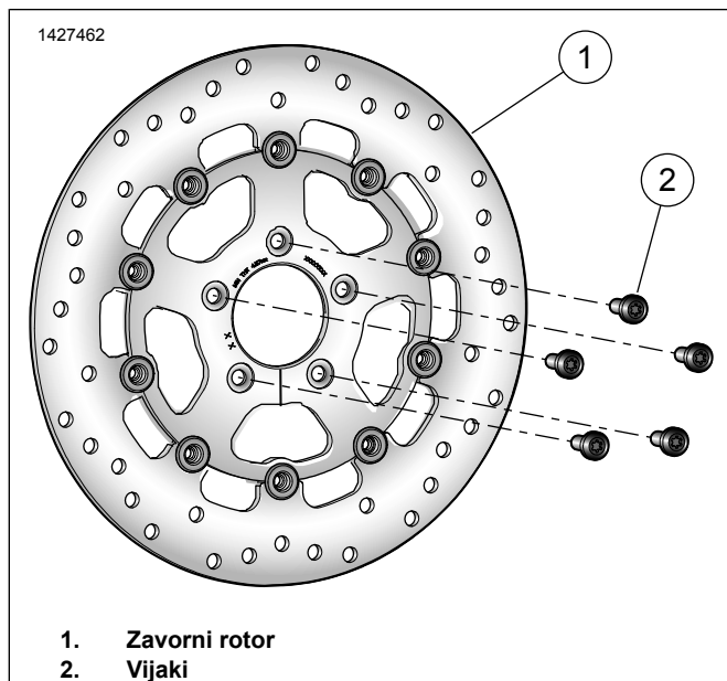
Slika 1. Servisni deli: Kompleti zadnjega zavornega rotorja (diska)
