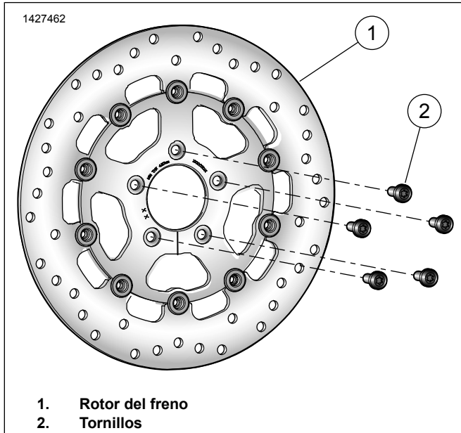
Figura 1. Piezas de servicio: Kits del rotor del freno trasero (disco)
