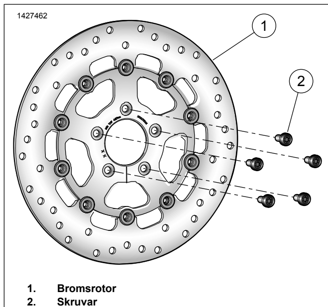
Figur 1. Reservdelar: Bakbromsrotorsatser (skivor)
