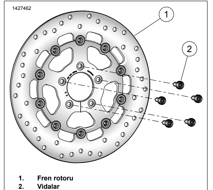
Şekil 1. Servis Parçaları: Arka Fren Rotoru (Diski) Kitleri
