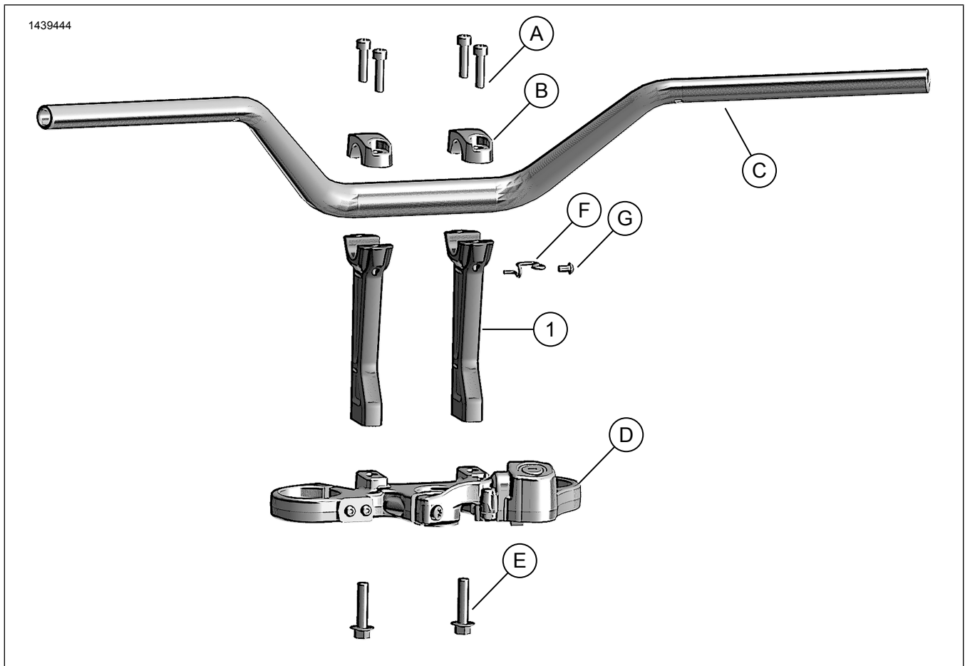
Figure 1. Liste des pièces de rechange : Kit supports de guidon hauts
