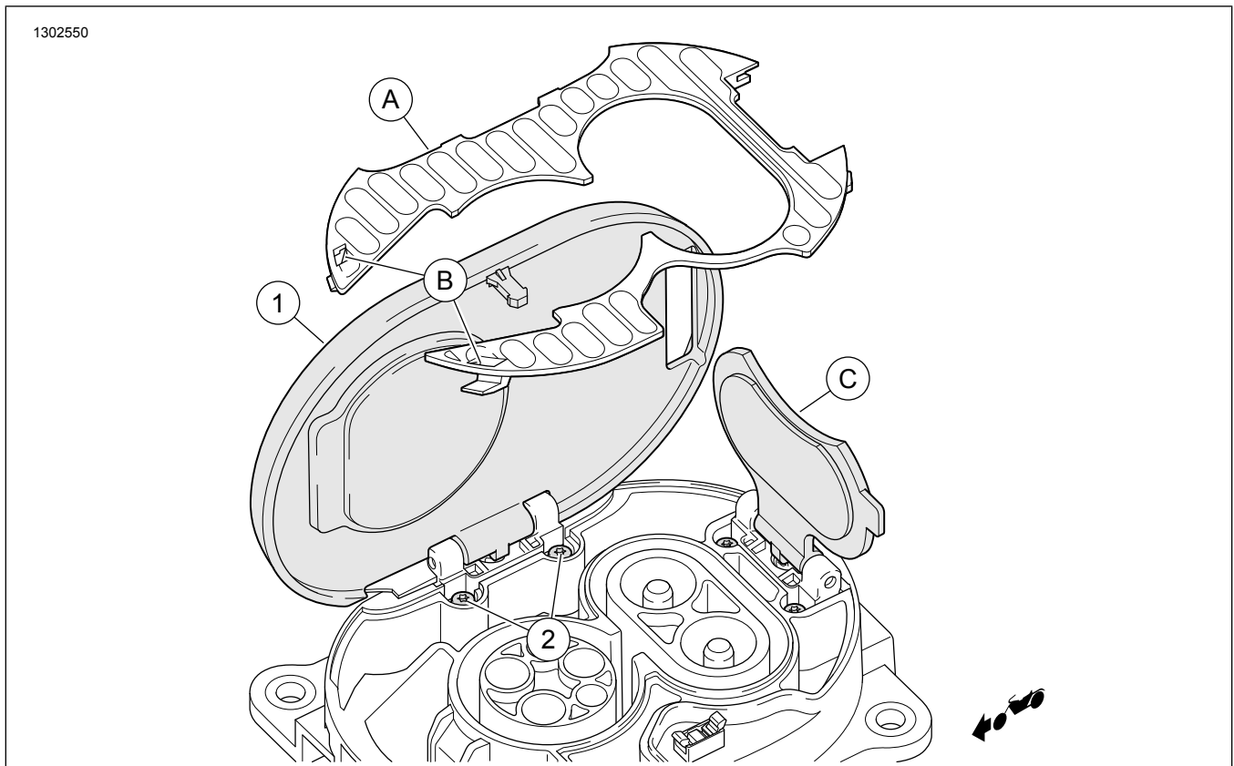
Figure 1. Contenu du kit : Porte de charge
