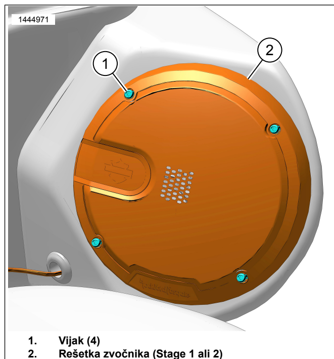
Slika 2. Rešetka podstavka zvočnika (prikazana je leva stran)
