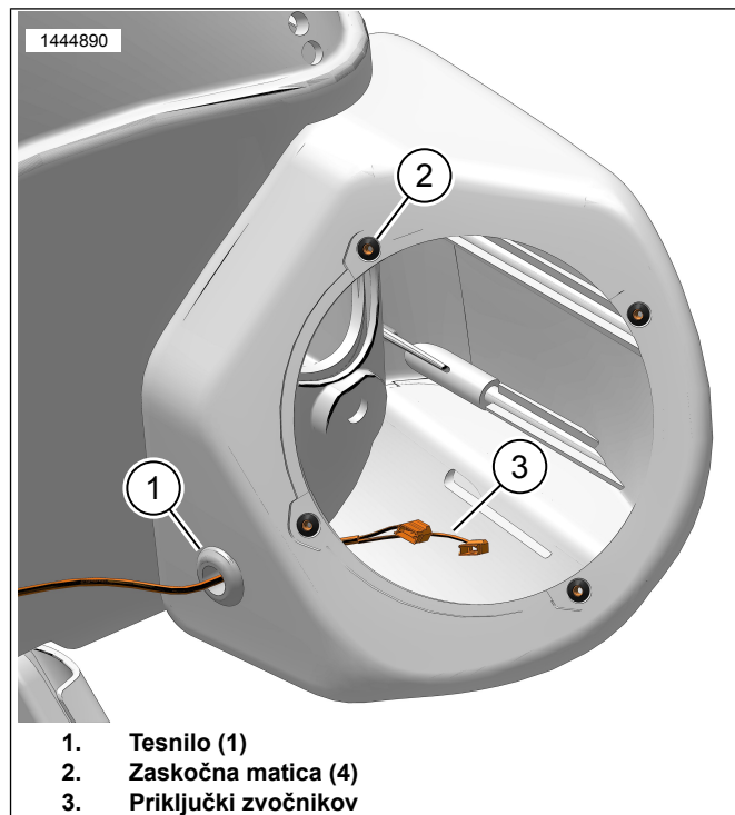
Slika 1. Kabelski snop podstavka zvočnika (prikazana je leva stran)
