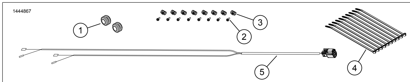
Slika 3. Nadomestni deli, zvočniki v spodnjem oklepu
