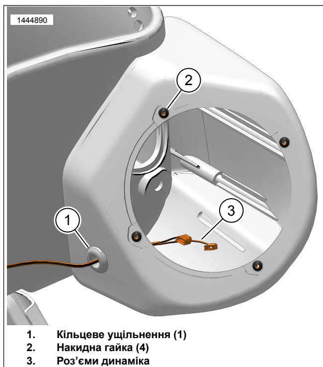
Малюнок 1. Джгут відсіку динаміка (показано ліву сторону)
