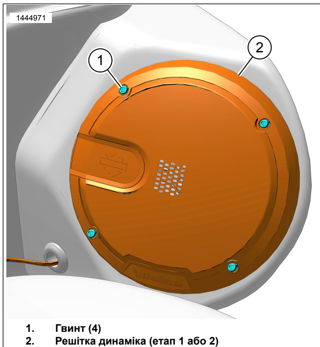
Малюнок 2. Решітка відсіку динаміка (показано ліву сторону)
