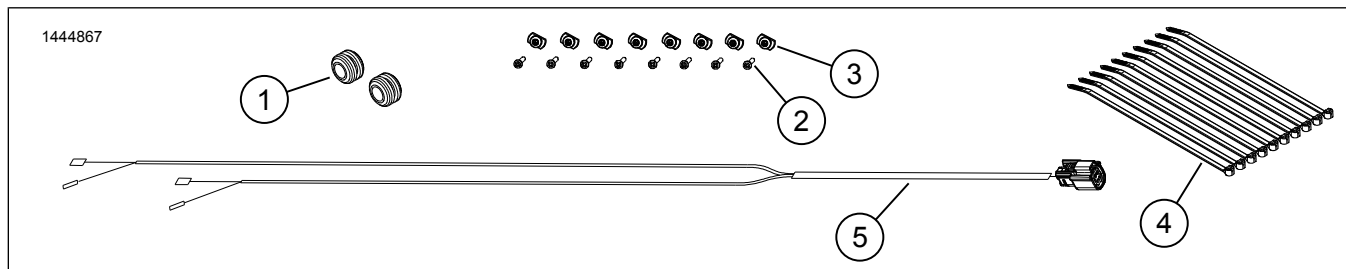
Slika 3. Servisni dijelovi, zvučnici u donjoj maski
