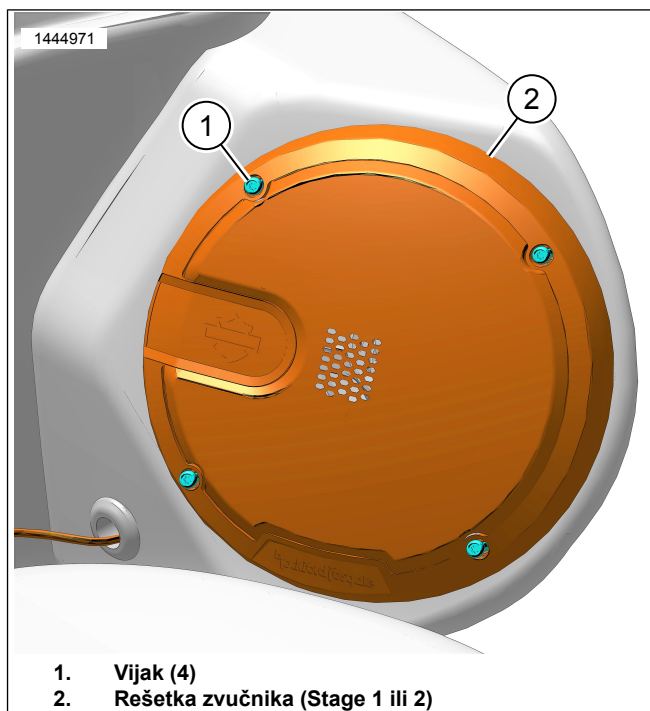
Slika 2. Rešetka zvučnika u kućištu (prikazana lijeva strana)
