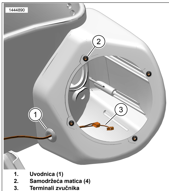
Slika 1. Kabelski snop zvučnika u kućištu (prikazana lijeva strana)
