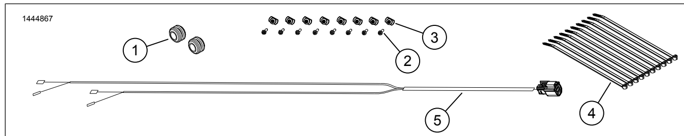
Joonis 3. Varuosad, gondli alaosa kõlarid
