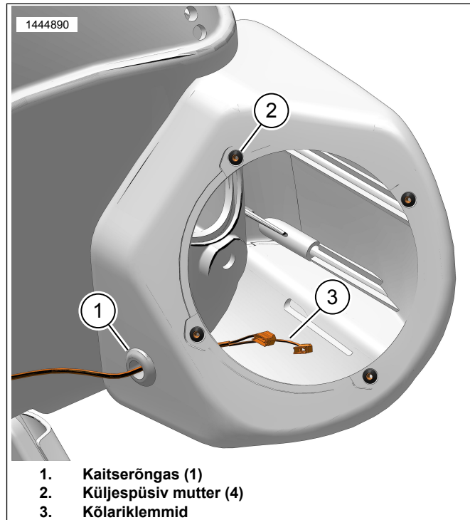
Joonis 1. Kõlaripodi juhtmestik (näidatud vasakpoolne)
