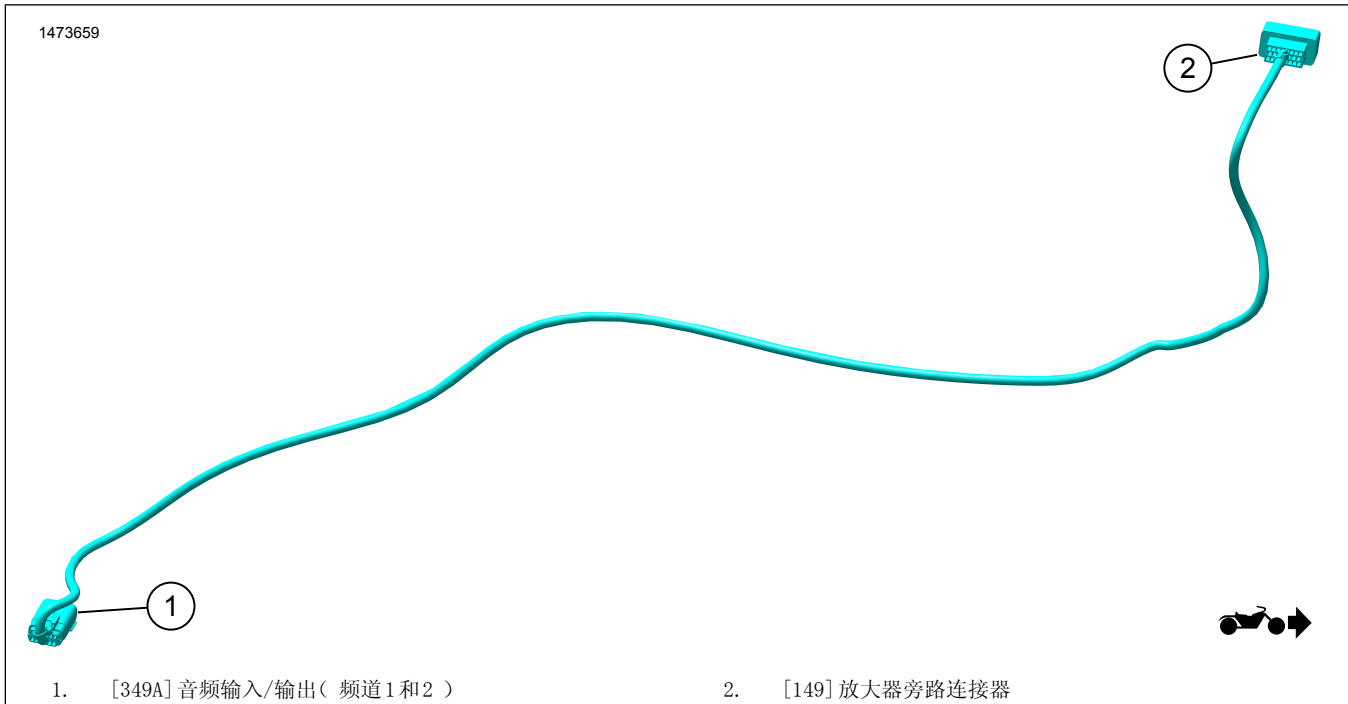
图1。挡风板扬声器线束
