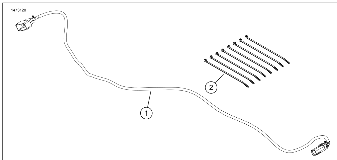
Slika 3. Servisni dijelovi, komplet za ugradnju pojačala
