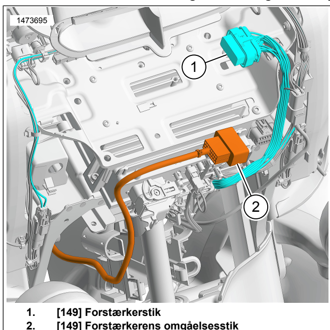
Figur 2. Gaffelmonteret strømlinebeklædning er vist, fast strømlinebeklædning er magen til
