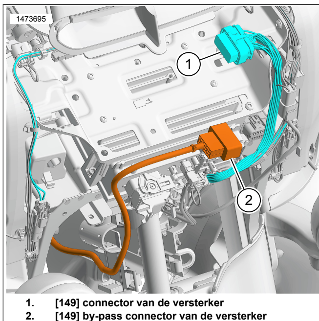
Afbeelding 2. Op de voorvork gemonteerde kuuip getoond, vergelijkbare bevestigde kuuip
