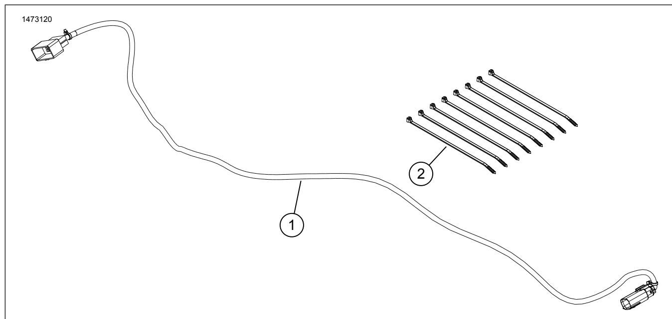
Afbeelding 3. Serviceonderdelen, versterkermontageset
