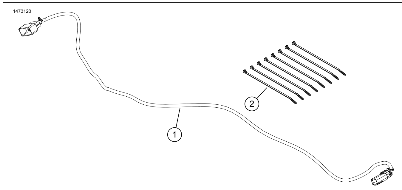
Joonis 3. Varuosad, võimendi paigalduskomplekt
