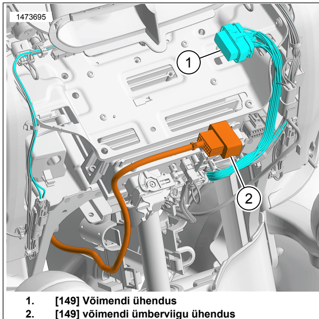
Joonis 2. Näidatud kahvlile paigaldatud gondel, fikseeritud gondel on sarnane
