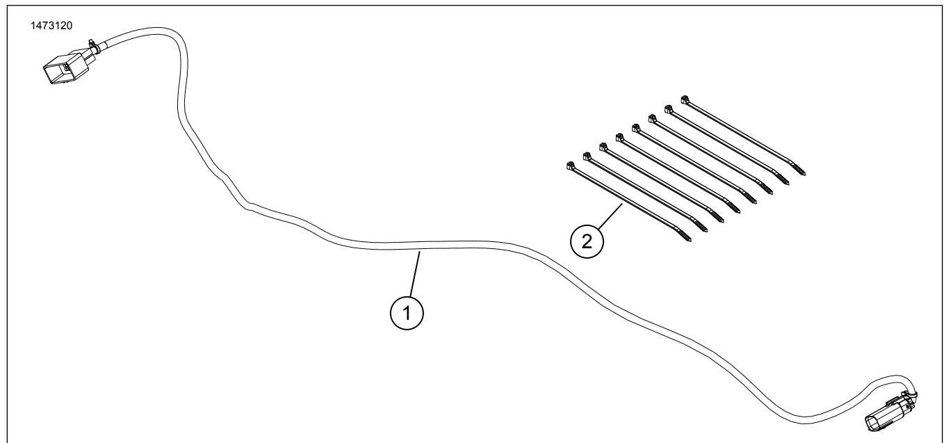
Kuva 3. Varaosat, vahvistimen asennussarja
