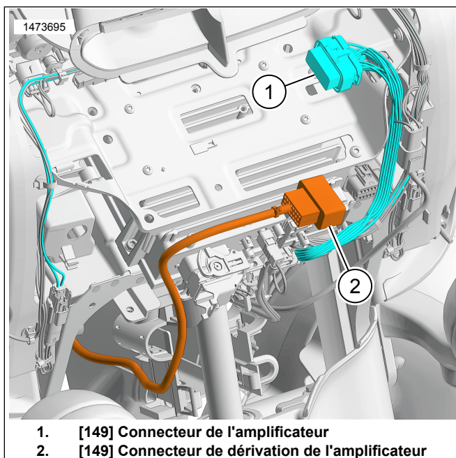
Figure 2. Carénage monté sur fourche représenté, carénage fixe similaire
