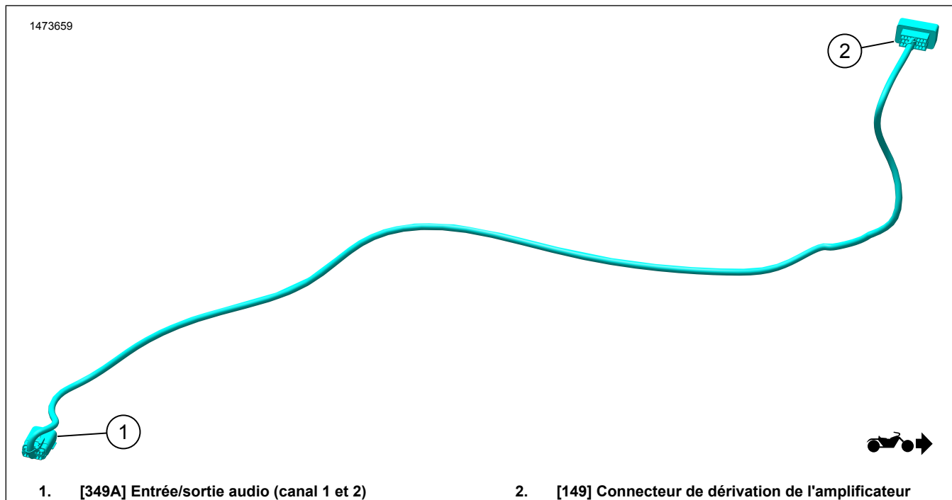
Figure 1. Faisceau haut-parleur de carénage
