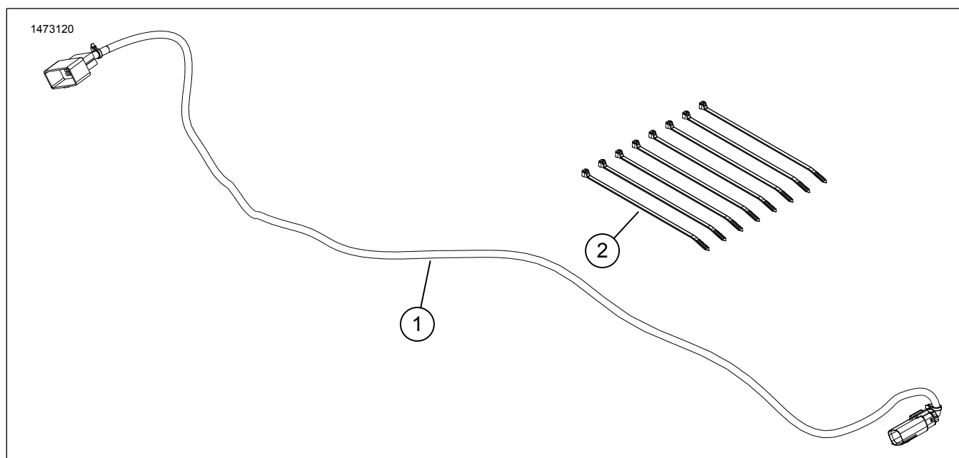
Figure 3. Pièces de rechange, kit d'installation d'amplificateur
