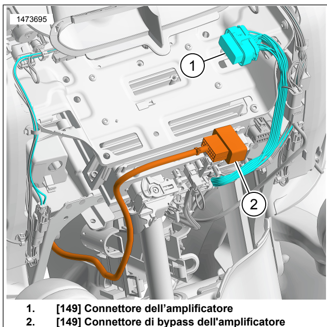
Figura 2. Illustrata: carenatura montata sulla forcella, simile per carenatura fissa
