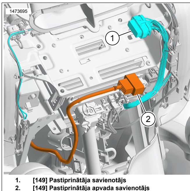
Attēls 2 Pie dakšas stiprināts aptecētājs parādīts, nostiprinātam aptecētājam līdzīgi
