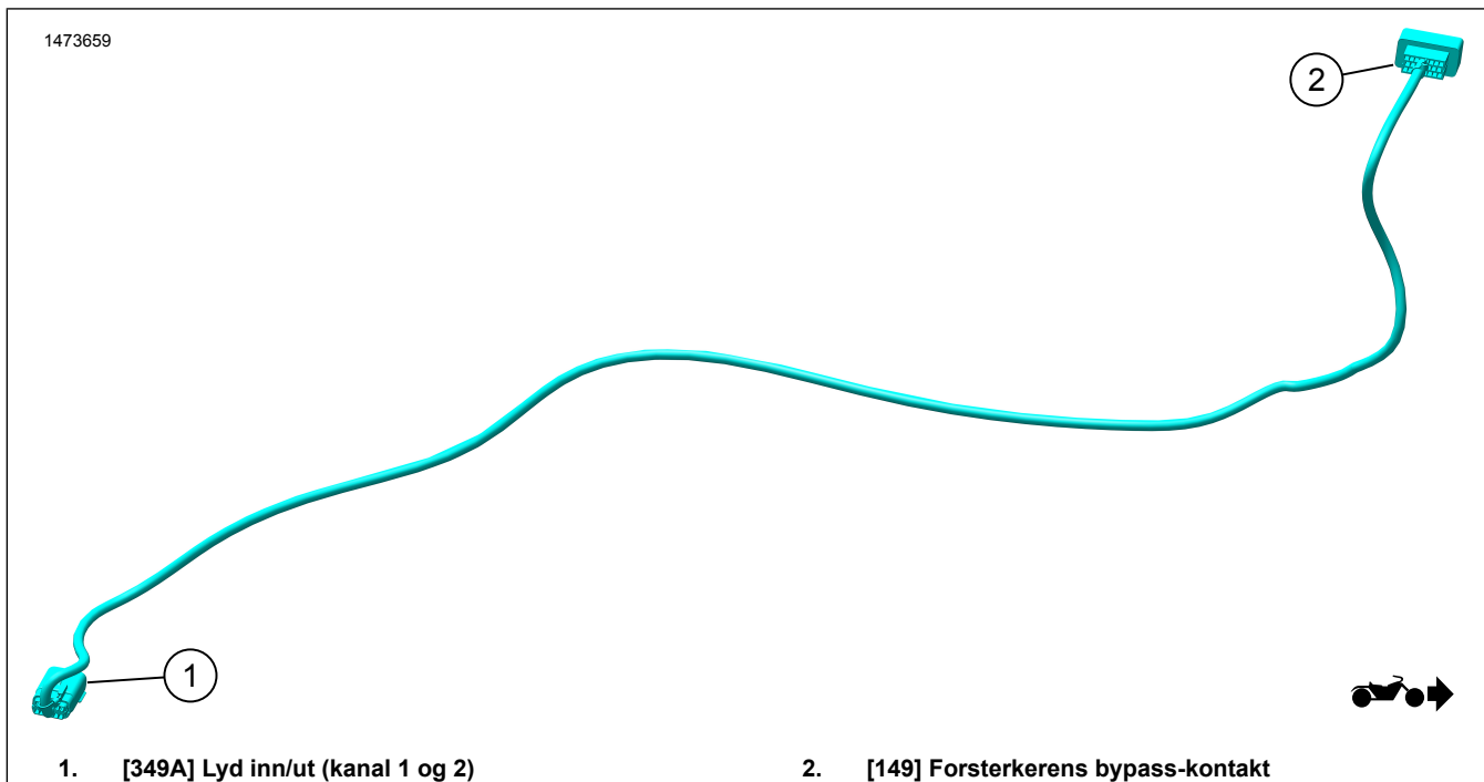
Figur 1. Ledningsnett til kåpehøytalere
