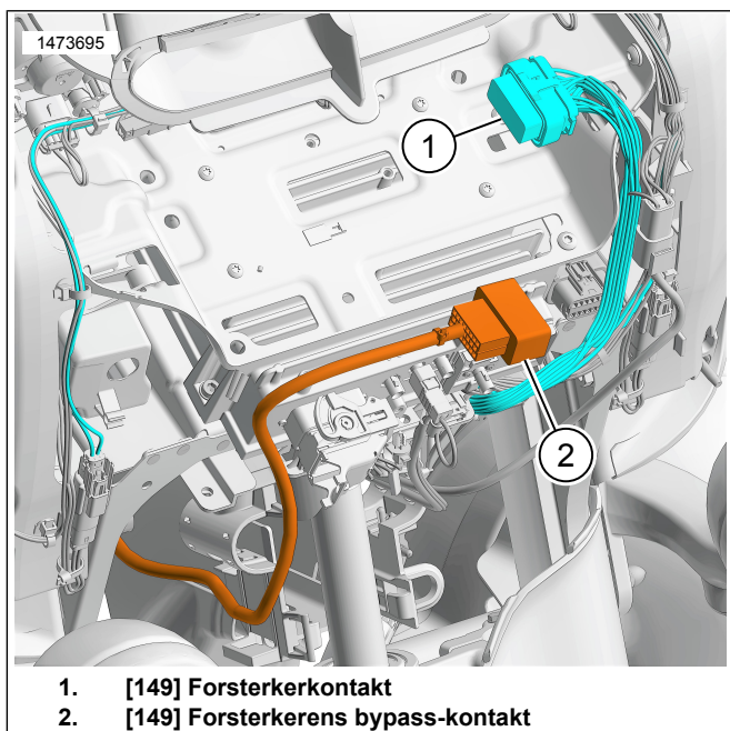
Figur 2. Gaffelmontert kåpe vist, fast kåpe er tilsvarende
