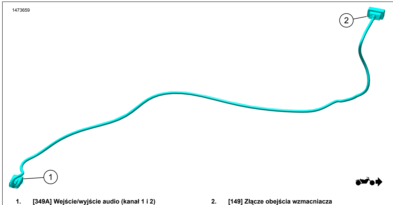
Rysunek 1. Wiązka głośników w owiewkach
