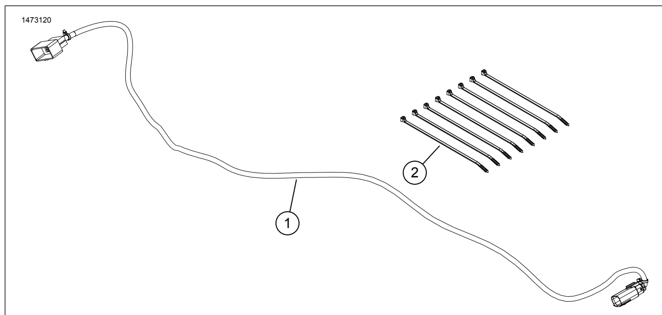
Figura 3. Kit de instalare amplificator, componente de service
