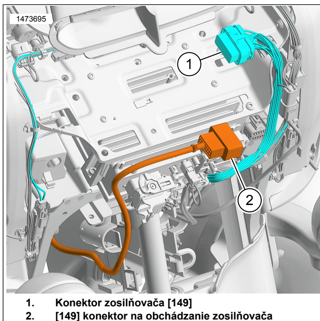
Obrázok 2. Zobrazená kapotáž upevnená na vidlici, pevná kapotáž je podobná
