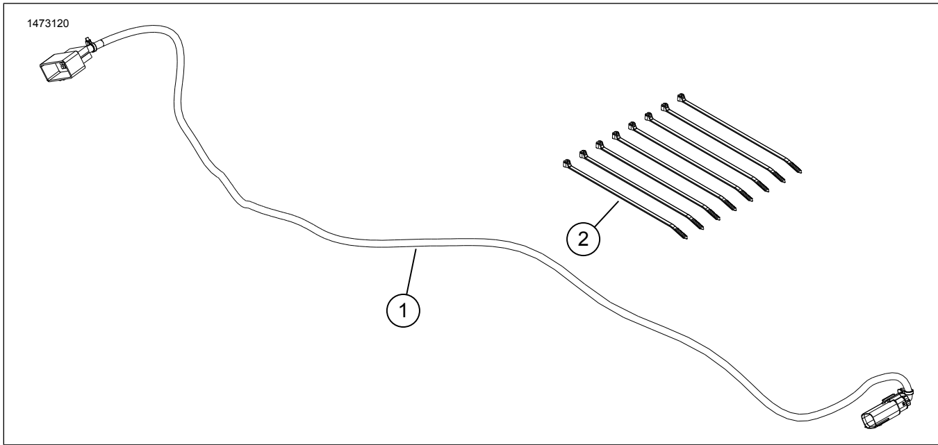
Figura 3. Piezas de servicio, Instalación del kit del amplificador
