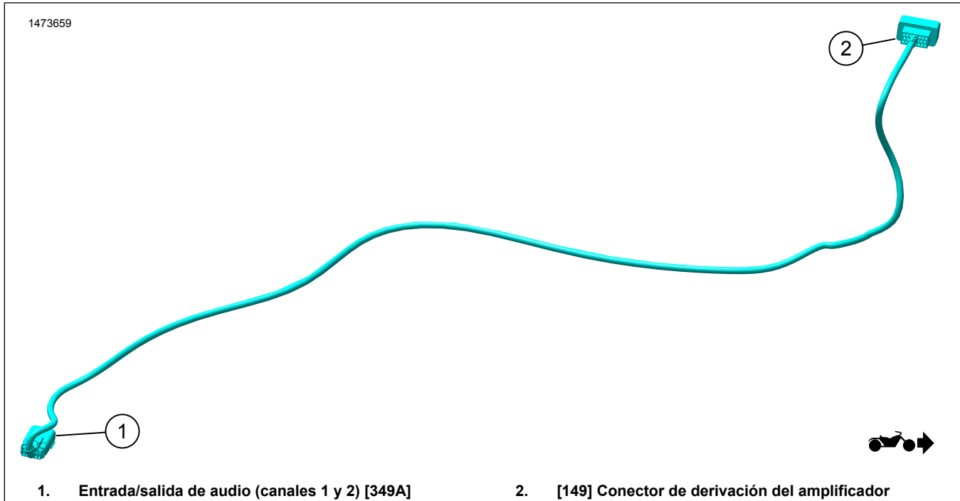
Figura 1. Arnés del altavoz en el fuselaje
